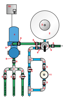
Filtration avec doseur de chlore en ligne
