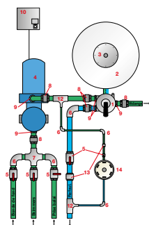
Filtration avec doseur de chlore en dérivation
